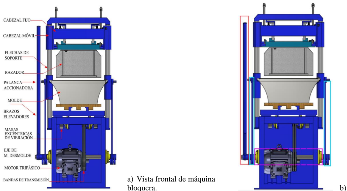
Figura 1. Máquina Bloquera Ponedora Manual en su modelo mecánico.
