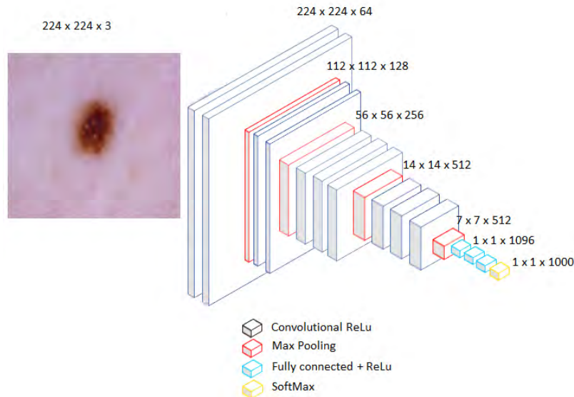
Figura 2. Arquitectura de la red convolucional VGG16 (ICHI.PRO, 2021).
