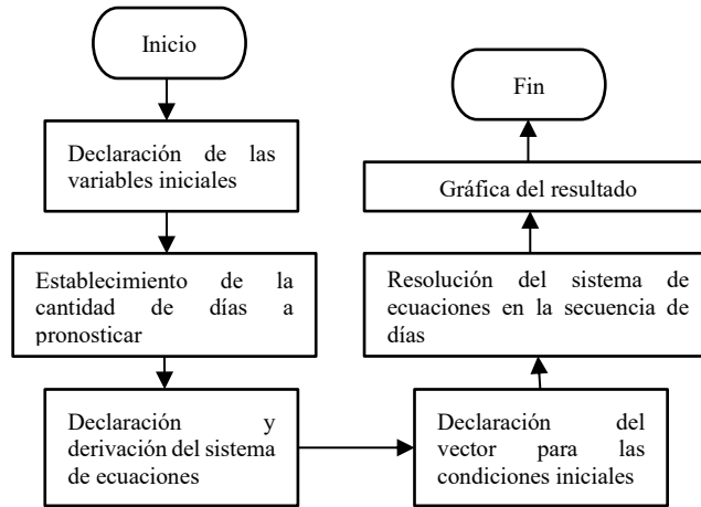
Figura 4 Diagrama de flujo para programación del algoritmo SIR.
