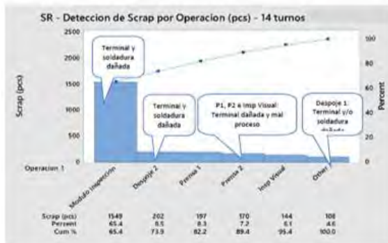
Figura 6. Análisis de Pareto Área SR por operación
