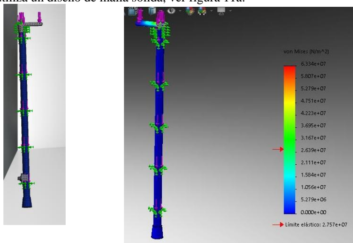
Figura 11. Mallado del modelo (11a) y Tensión de Von Mises (11b).
