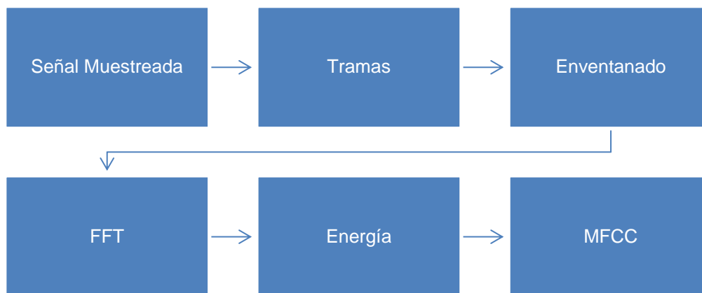
Figura 1. Etapas de procesamiento de la señal para los fonemas.
