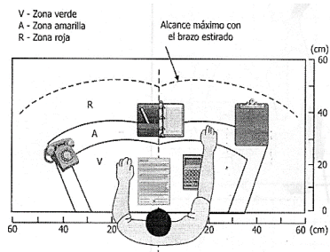
Fig.1 Límites de alcance en el plano horizontal.
