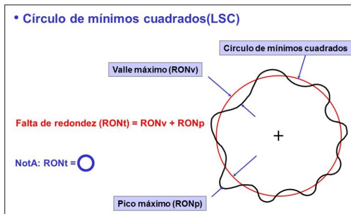
Fig. 1 esquema de LSC [1]
