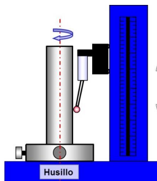
Figura. 4 Husillo eje de referencia giratorio
