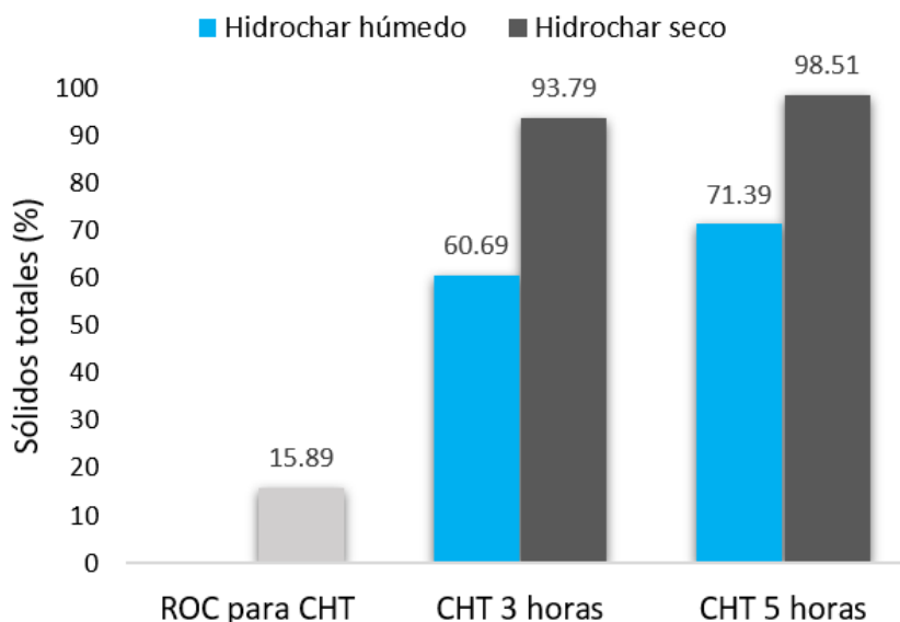
Figura 6. Resultados de porcentaje de sólidos totales.
